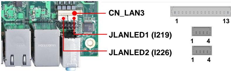
CN_LAN3: 13-pin i226-LM connector
